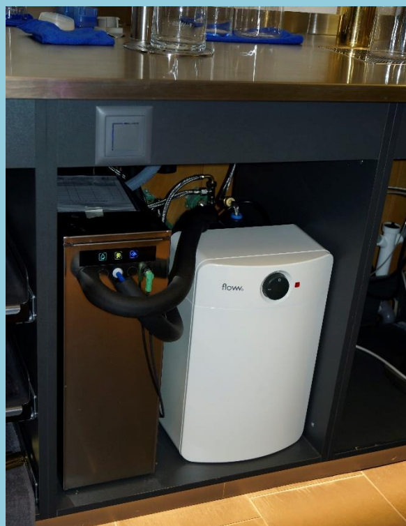
UT40HCS Gastro mit 10 Liter Boiler
