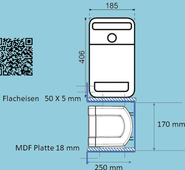
Wand Doppel Konsole für HCS
